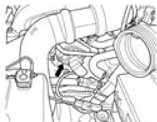
Fig. 1 Camshaft Position Sensor - 2.0L 4L DOHC
