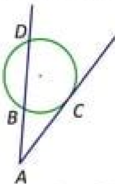
Secant-Tangent
